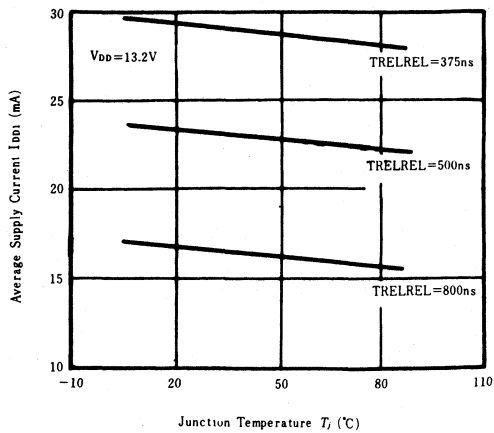
IDD1 vs. T_j
