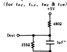
Output Load B
